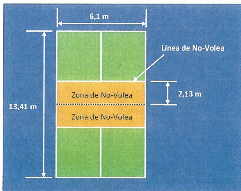
Dimensiones de la Pista de Pickleball
